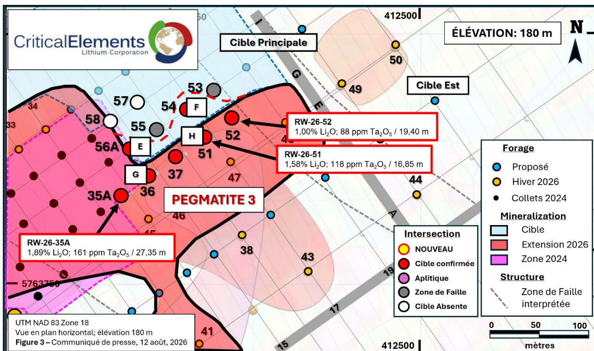
Figure 3: Projection en plan de la Pegmatite 3 – Contours de la zone et des extensions ciblées.
